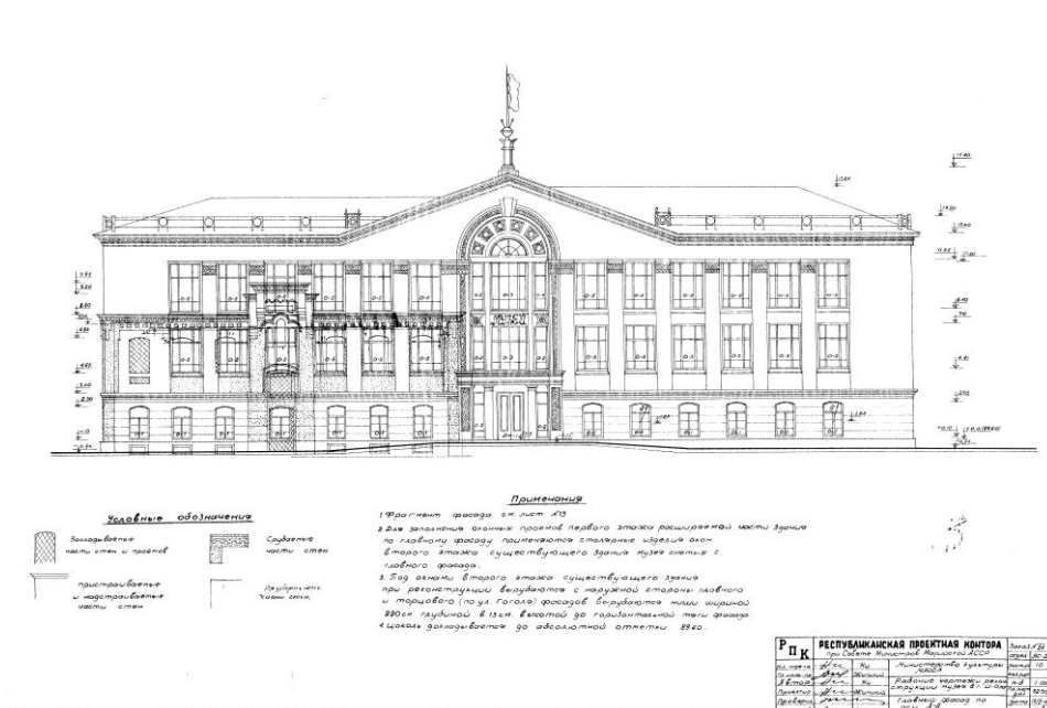
Проект реконструкции здания музея. 1960 г. Архив АО «Марийскгражданпроект – базовый территориальный проектный институт». Л. 10.
